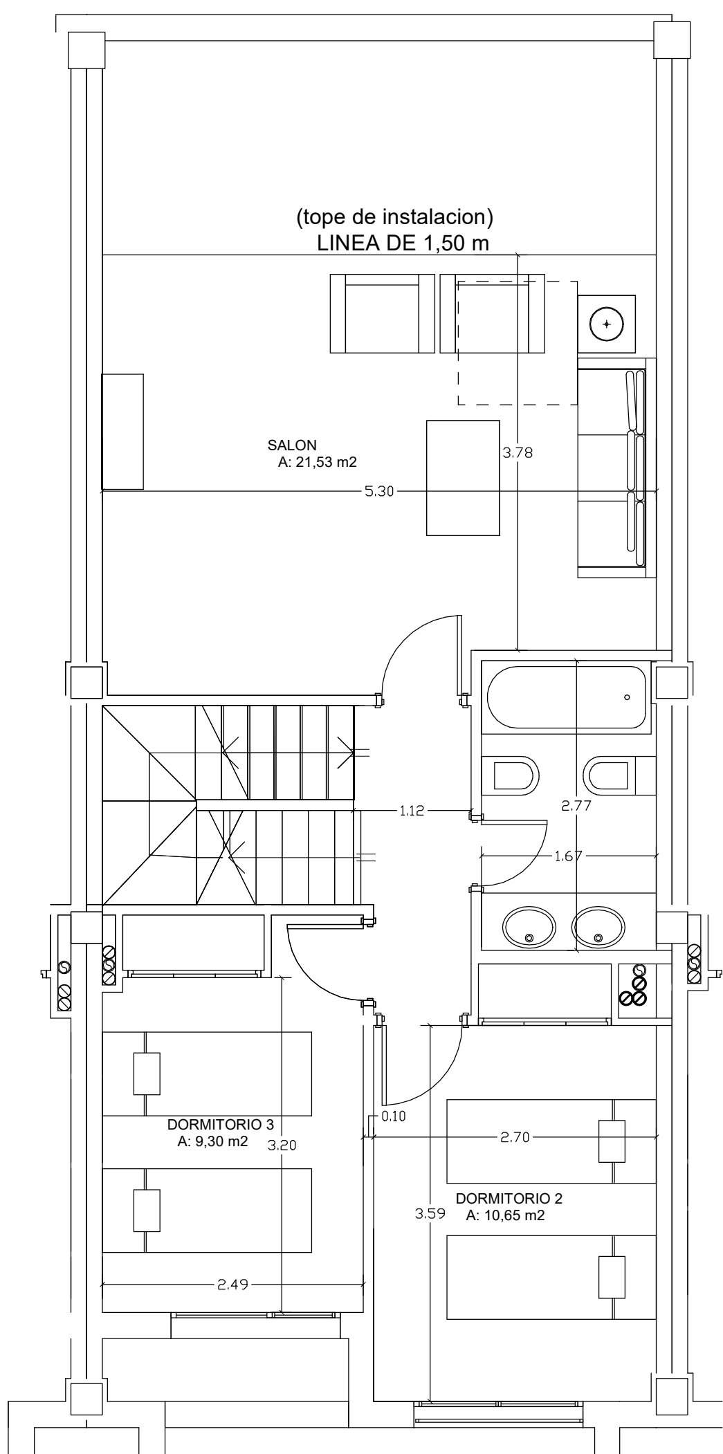
PLANTA 2º
